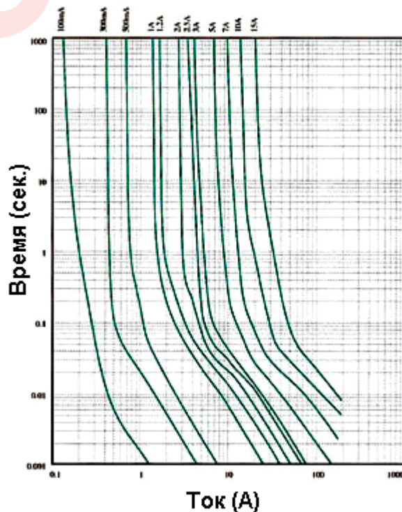
Токовременная зависимость
