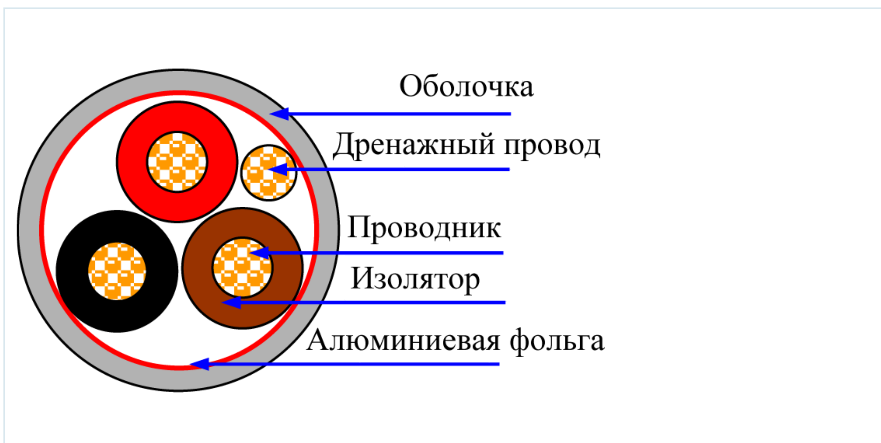
Схема изделия
