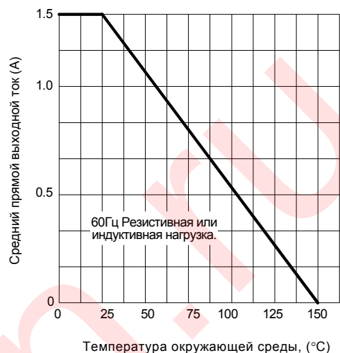
Рис.2 - График снижения выходного тока
