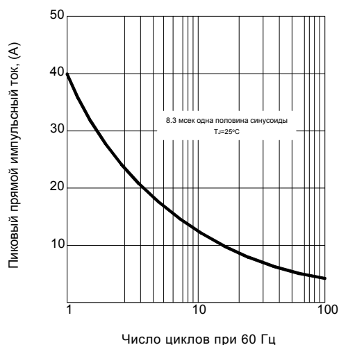
Рис.1 - Максимальный неповторяющийся пиковый ударный прямой ток
