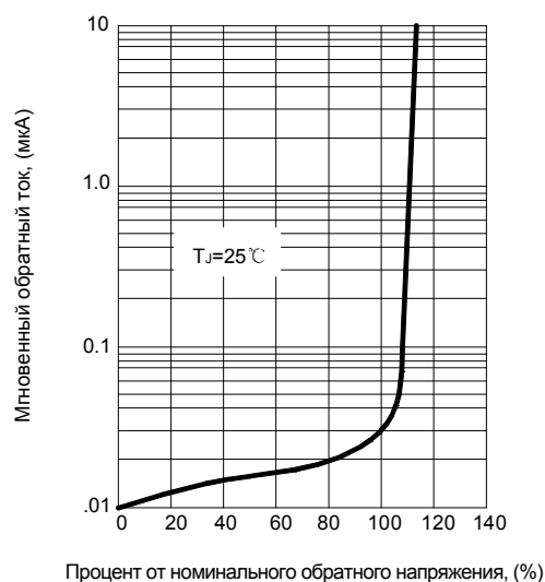
Рис.4 - Типичная обратная характеристика
