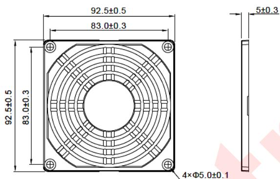
УМ-09 Для 92мм вентилятора
