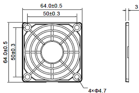
УМ-06 Для 60мм вентилятора
