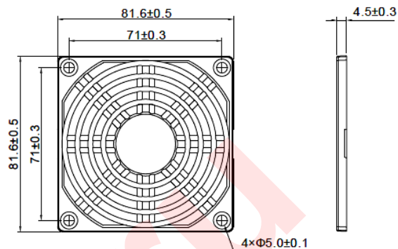
УМ-08 Для 80мм вентилятора
