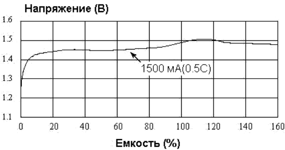
Быстрый заряд (требуемое управление зарядом)
