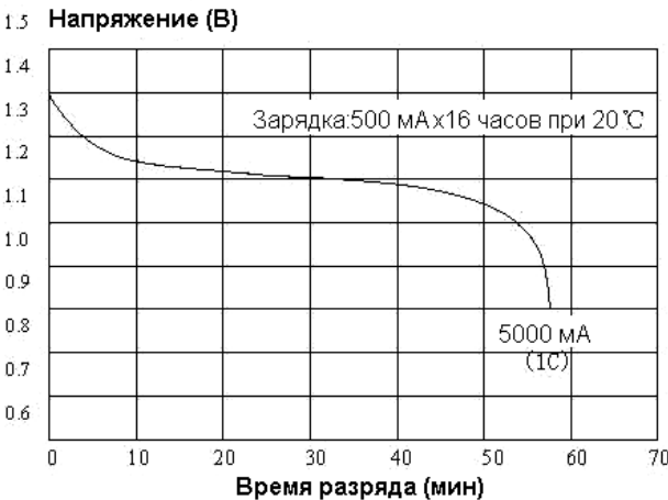
Высокая скорость разряда
