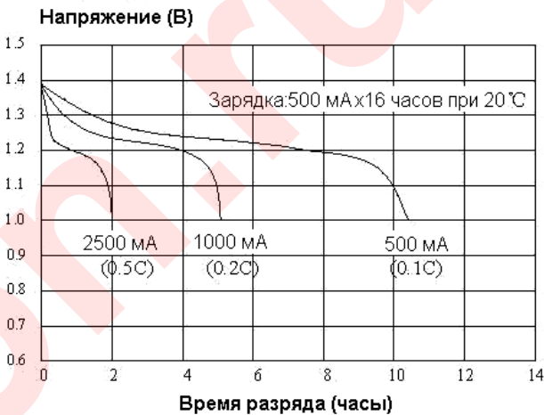
Низкая скорость разряда
