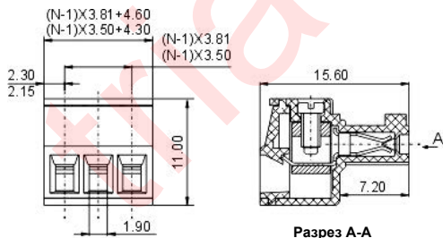
Разрез А-А
