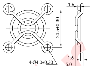
FG-03 для 30 мм вентилятора
