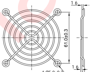
FG-07 для 70 мм вентилятора
