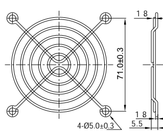
FG-08 для 80 мм вентилятора
