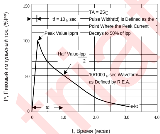
Рис.3 - Форма импульса
