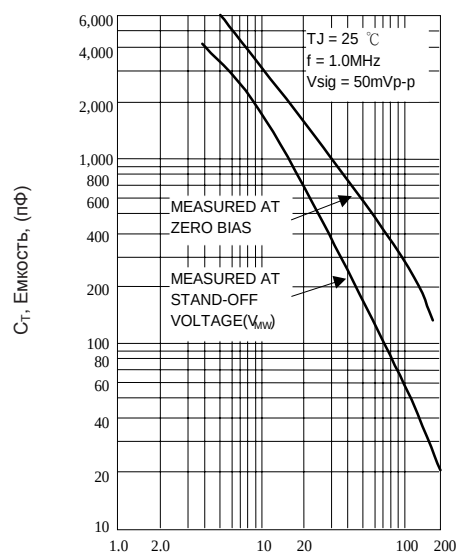
Рис.4- Типичная общая емкость
