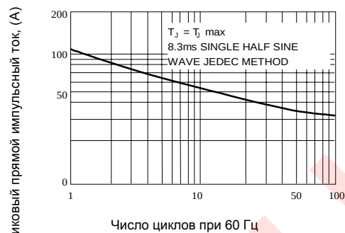
Рис.6 - Максимальный неповторяющийся пиковый ударный прямой ток
